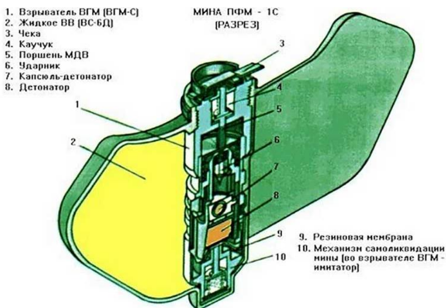
Рис. 3 – ПФМ-1 «Лепесток» 6 .
