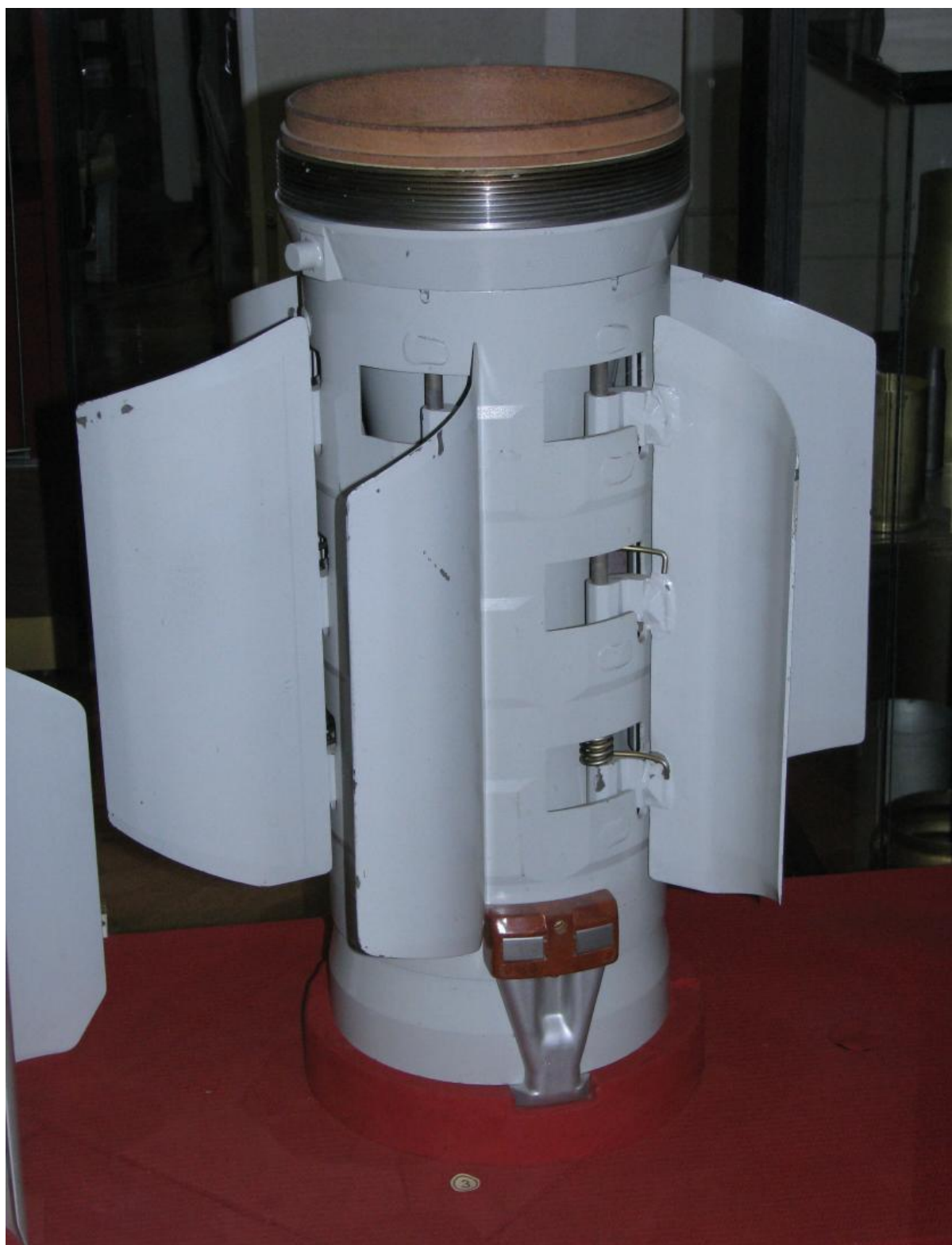
Рис. 29 - Макет блока стабилизатора для снаряда РСЗО «Смерч» 47 .
