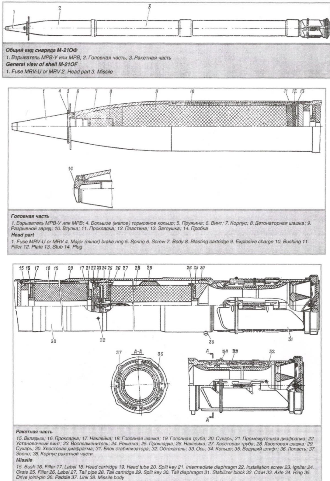
Рис. 34 - Конструкция снаряда М-21ОФ (осколочно-фугасный снаряд, применяемый для стрельбы из РСЗО 9К51 «Град» 52 ).
