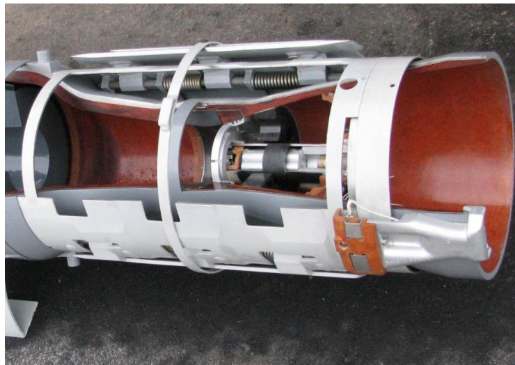
Рис. 28 - Вид хвостового блока разрезного макета снаряда для РСЗО «Смерч» 46 .
