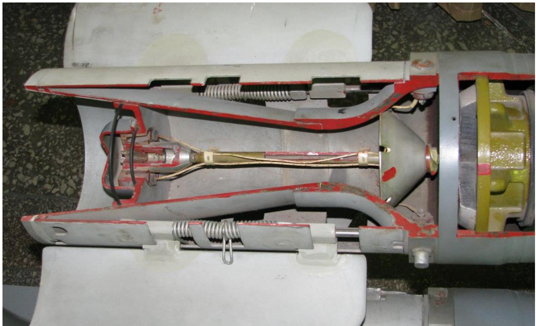
Рис. 31 – Вид хвостового блока разрезного макета снаряда РСЗО «Ураган» 49 .
