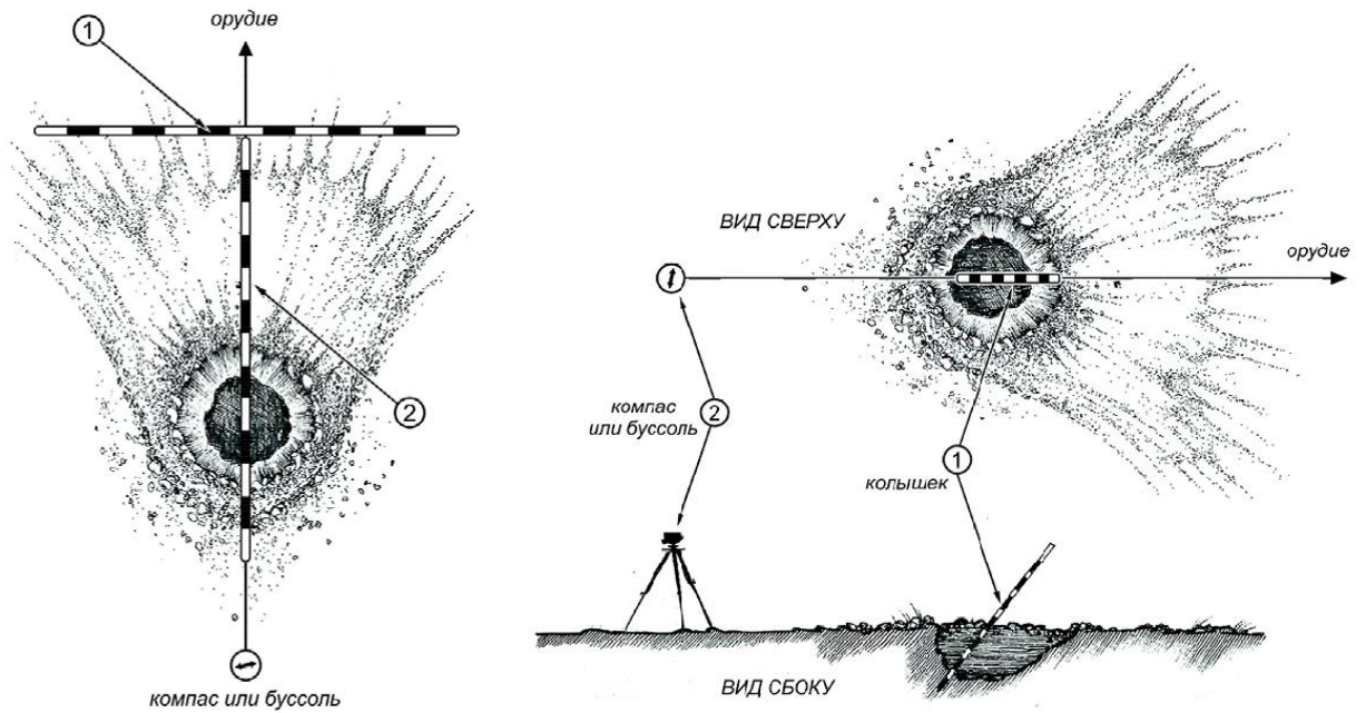
Рис. 25 – Методы определения направления обстрела: слева – метод осколочных канавок; справа – метод скважины взрывателя.
