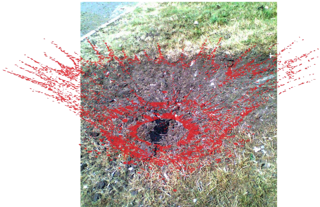
Рис. 24 – Попадание № 1: воронка соответствует форме воронки от обстрела снарядами под большим углом встречи.
