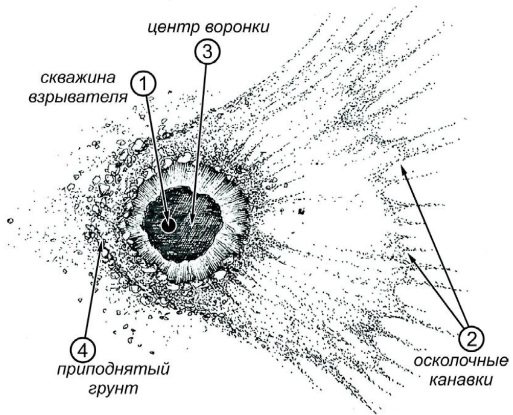
Рис. 23 – Воронка от снаряда, соприкоснувшись с поверхностью под большим углом встречи.
