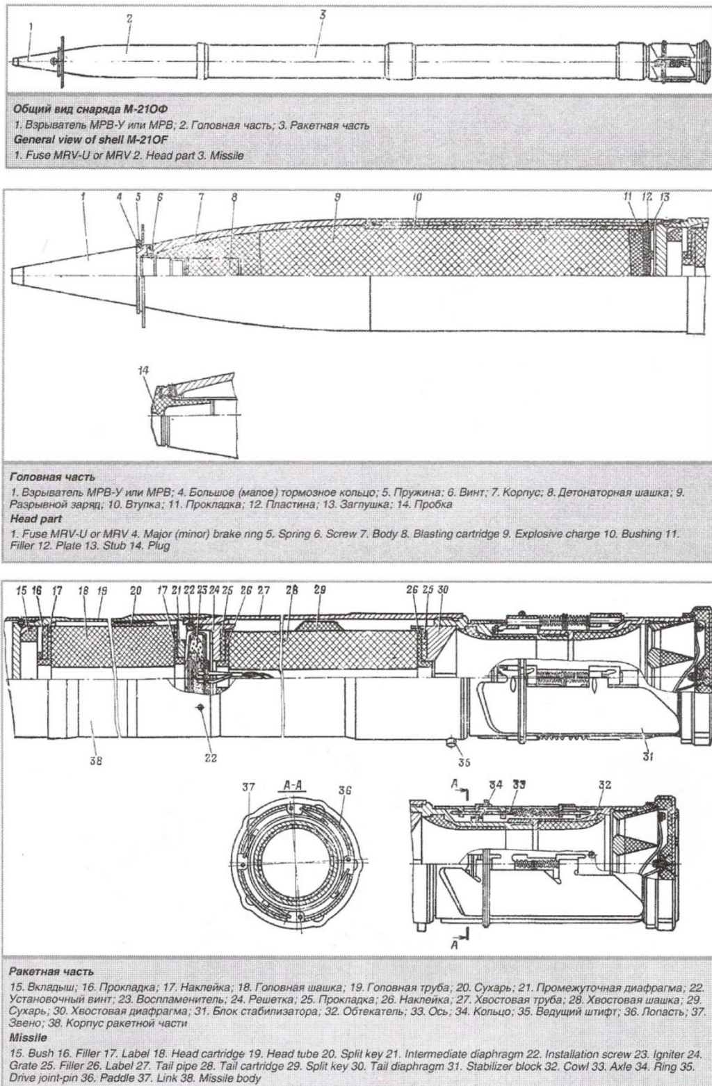
Рис. 27 - Конструкция снаряда М-21ОФ (осколочно-фугасный снаряд, применяемый для стрельбы из РСЗО 9К51 «Град»)²⁶.
